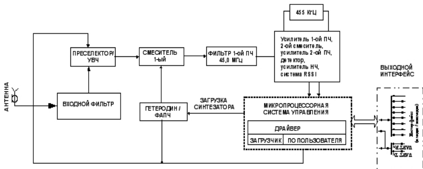
Структурная схема приемника RRx-450
